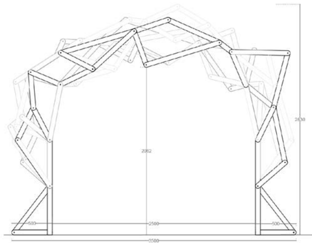
a.Elévation sur un module composé de 6 arches - 1/200è
